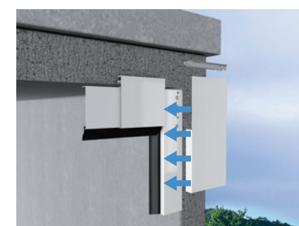
Universal-Blendlösung, Außenansicht
